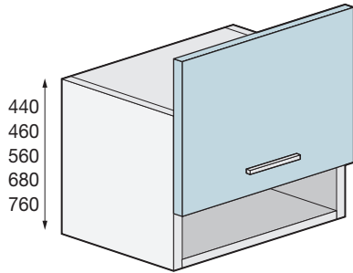
Height H. 440 mm - H. 460 mm H. 560 mm - H. 680 mm - H. 760 mm Inside space
