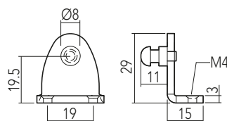
Attacco per telaio alluminio Joint for aluminium frame
