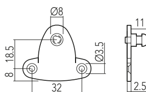
Attacco per telaio alluminio Joint for aluminium frame
